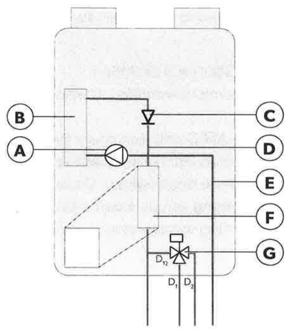
Figuur 8 Modul-AIR All-E
