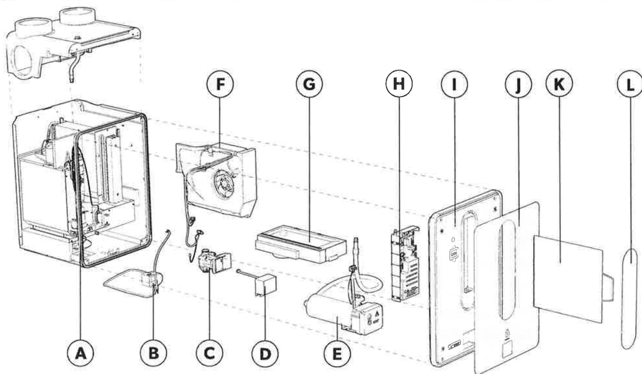
Figuur 4 Hoofdonderdelen van de Modul-AIR
