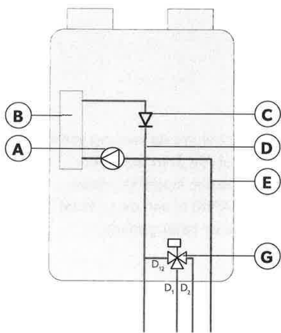
Figuur 7 Modul-AIR Combi
