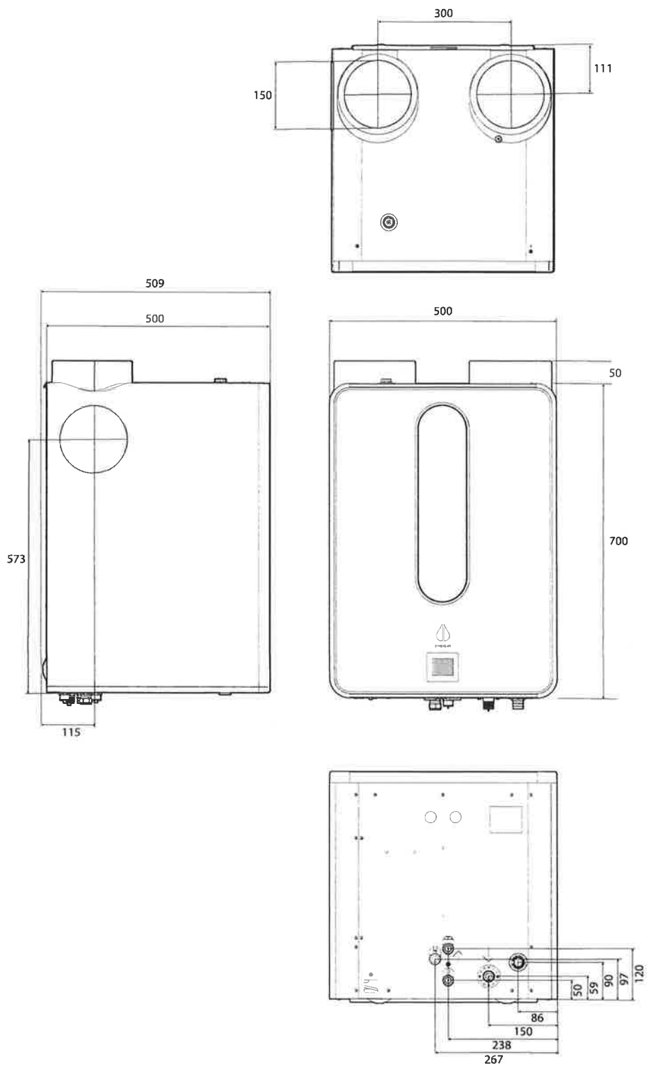
Figuur 20 De afmetingen van de Modul-AIR.
