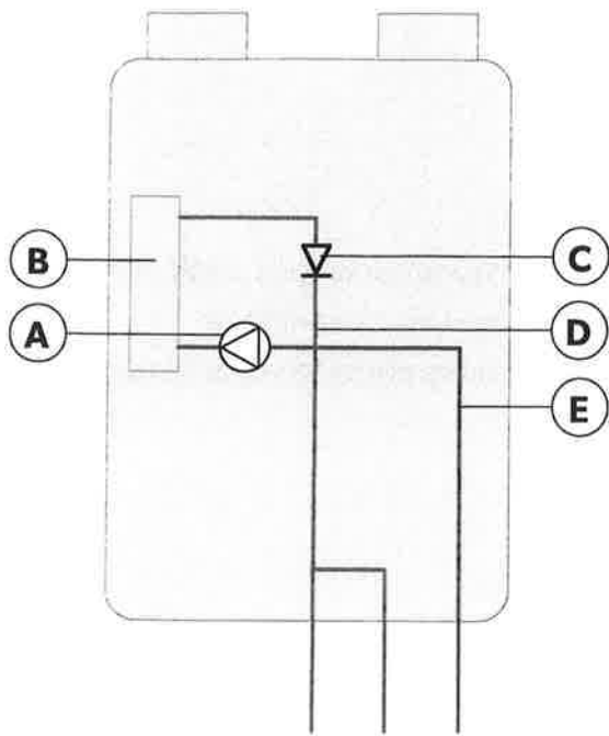
Figuur 5 Modul-AIR Solo
