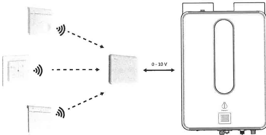
Figuur 13 Het draadloze bedieningsnetwerk van de Modul-AIR.
